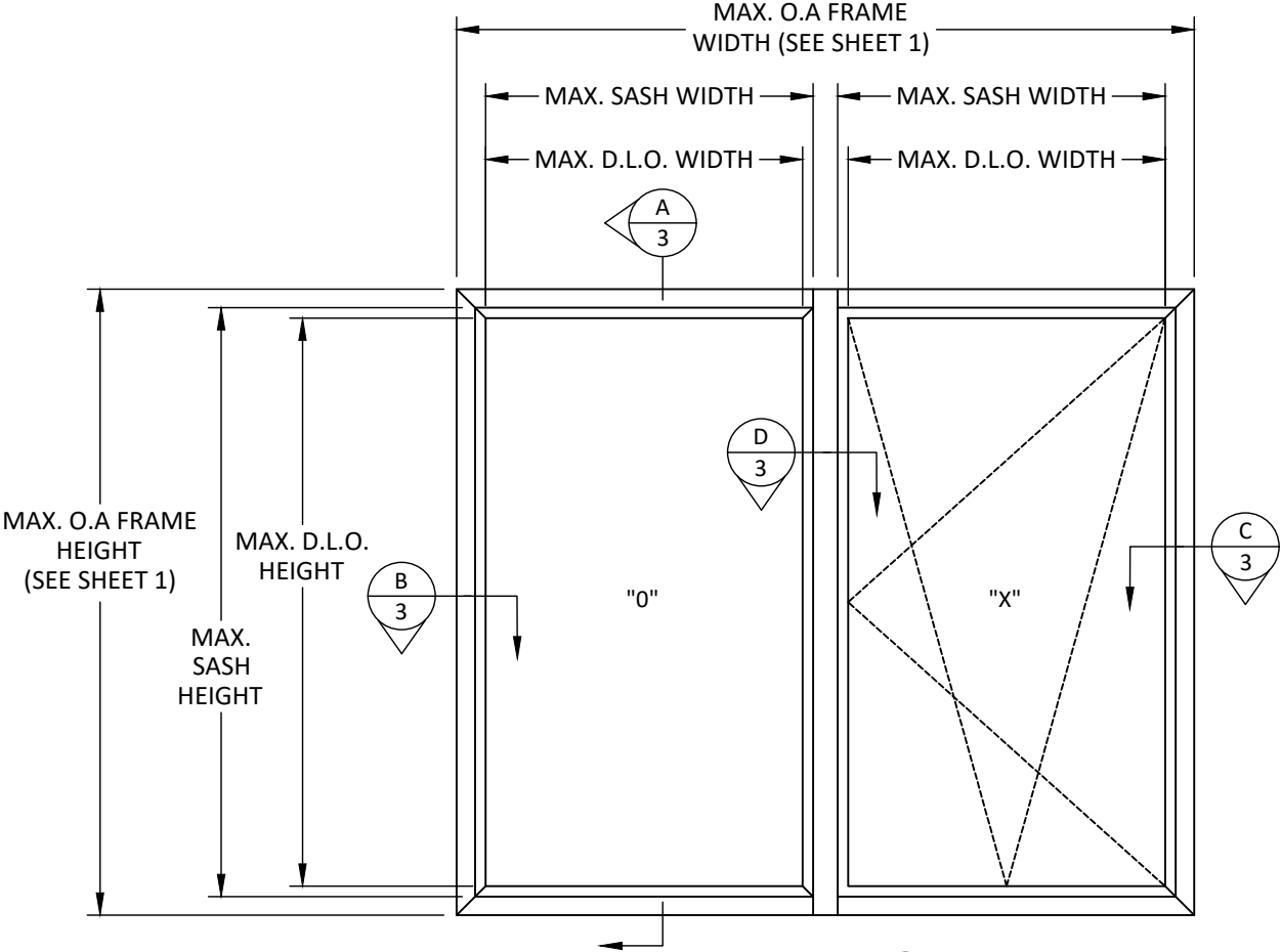
ELEVATION SLIDING & TILT PATIO DOOR
